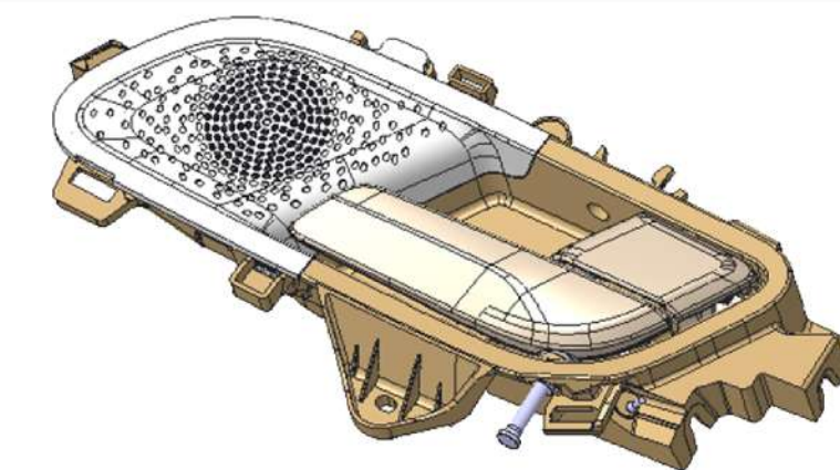
INNER DOOR HANDLE
